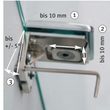
Wandwinkel innen (ohne Abdeckung)
