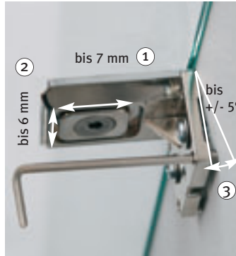
Wandwinkel außen (ohne Abdeckung)
