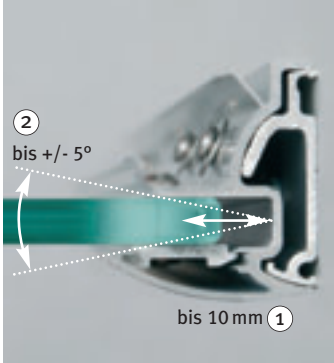
Wandprofilquerschnitt (ohne Abdeckung)
