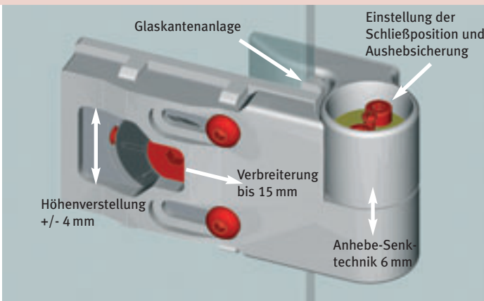
CAD-Darstellung ohne Abdeckung
