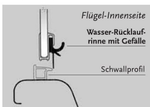
Ausführung SGw Pendel-Drehtüren mit Wasser-Rücklaufrinne unten (PVC) und Magnetprofile senkrecht (Alu).
