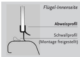
Ausführung SGA Pendel-Drehtüren mit Abweisprofil unten (PVC) und Magnetprofile senkrecht (PVC).
