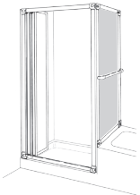
SL 31 mit SL/SF 65/66
